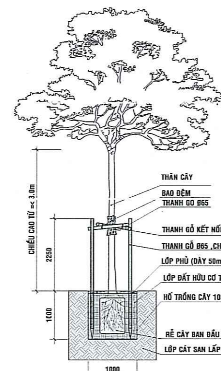
HỒ TRỒNG CÂY ĐIỂN HÌNH
