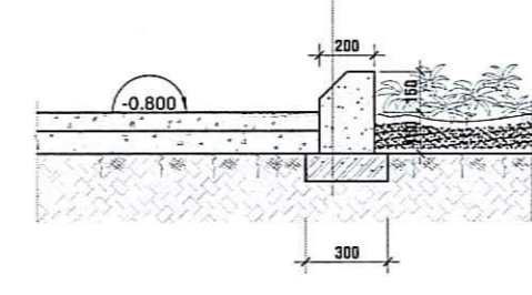
CHI TIẾT BÓ VỈA BÓN HOA
