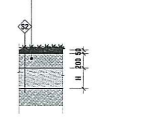
CHI TIẾT THÂM CỎ
