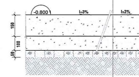
CHI TIẾT SÂN BÊ TÔNG
